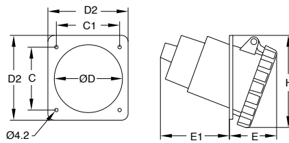
Ölçüler (mm)
