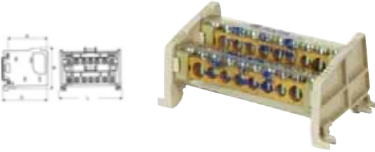
Ray Geniřlięi 35 KABLO KESİTİ 50mm 2
