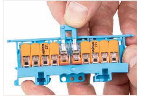
Köprüyü açık kelepçeleme birimlerinden çıkarın.
