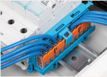
Kilitleme fonksiyonu ile: Kilitleme işlevine sahip köprü, ekeme konektörlerine takılır.
