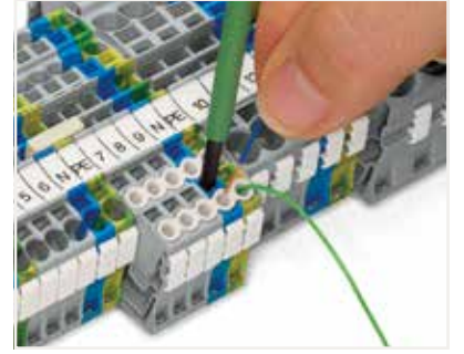
Yalıtım durdurucusuna bir iletken takın.
