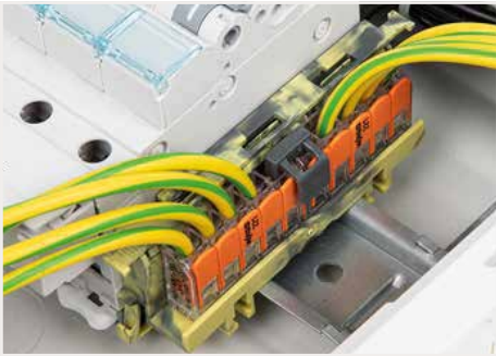
Kilitlelenebilir köprü, ekeme konektörlerine takılır.
